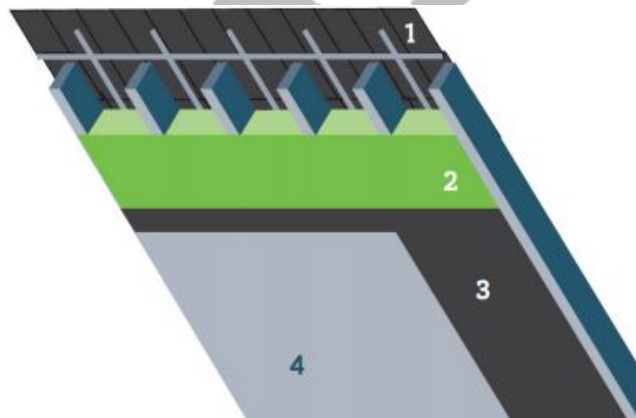
1. Onderdak | 2. Isolatie | 3. Damperscherm | 4. binnenafwerking
